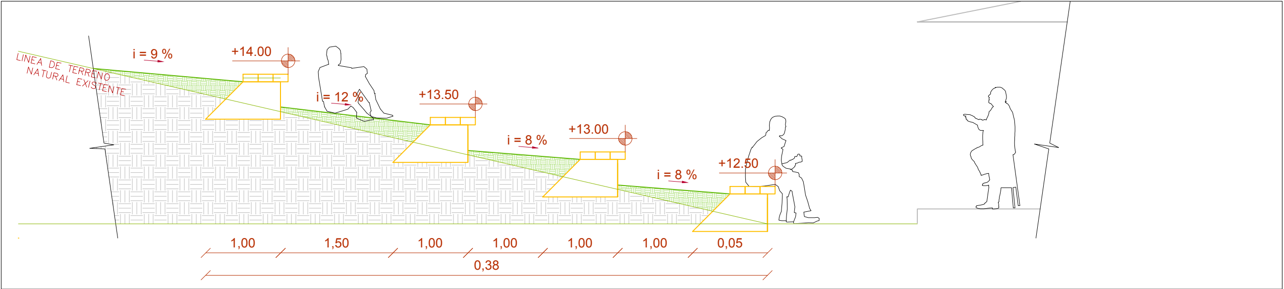
CORTE GAVIONES 1:50
