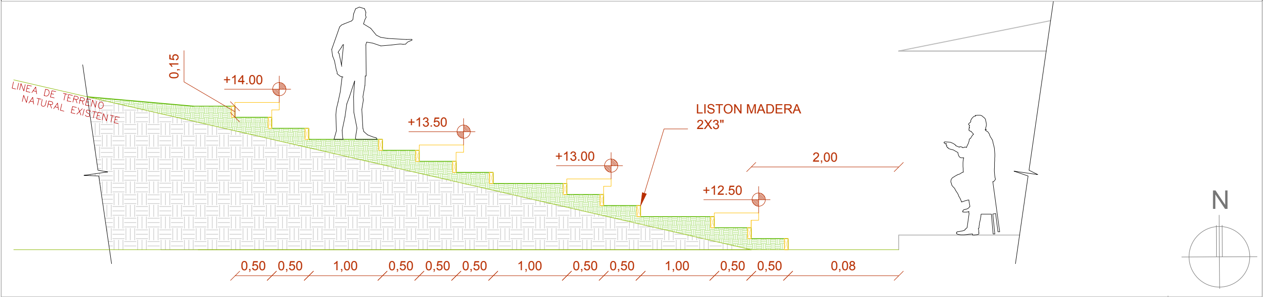
CORTE ESCALERA ANFITEATRO 1:50
